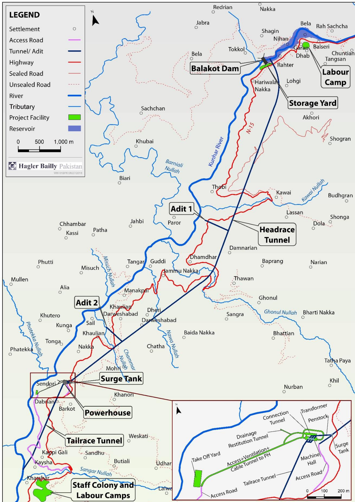
شکل نمبر 2: ہائیڈرو پاور ڈویلپمنٹ انویسٹمنٹ پراجیکٹ کی تفصیلات کا خاکہ
